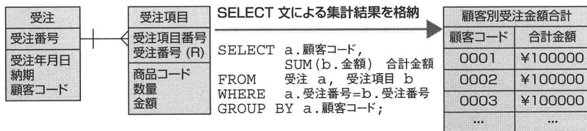
図 23 マテリアライズドビュー
